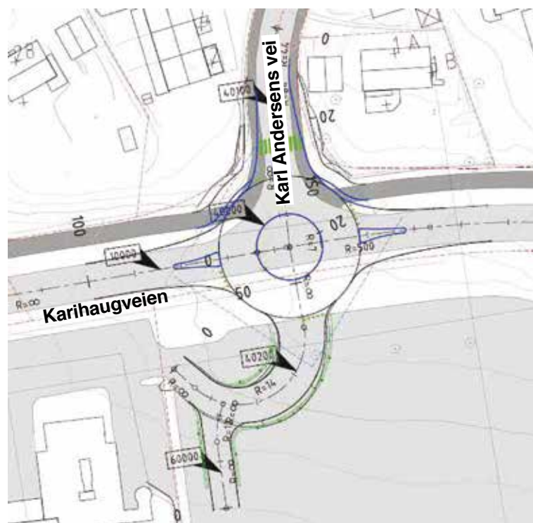
Utforming av rundkjøring i krysset Karihaugveien/Karl Andersens vei. (Kilde: Multikonsult.)
